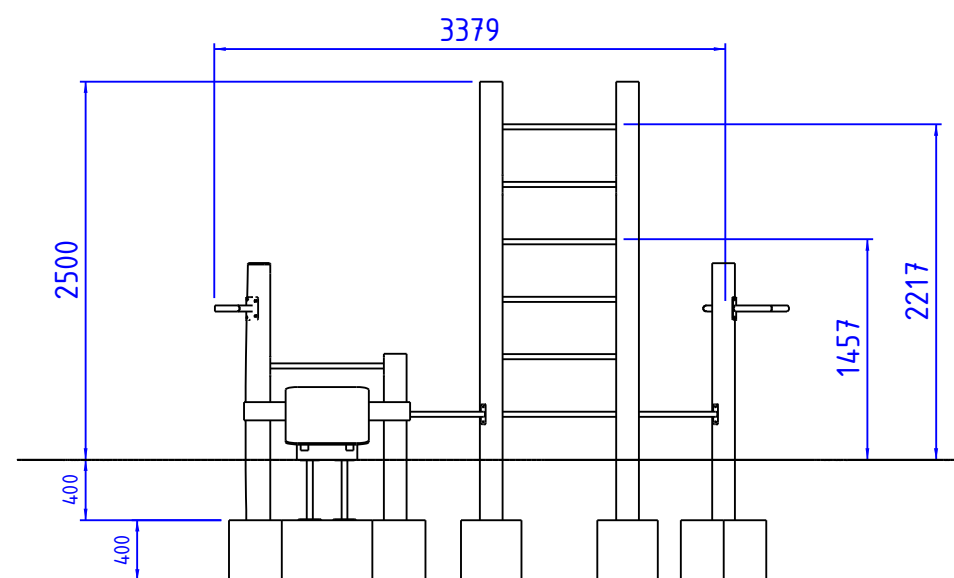
Vue face
