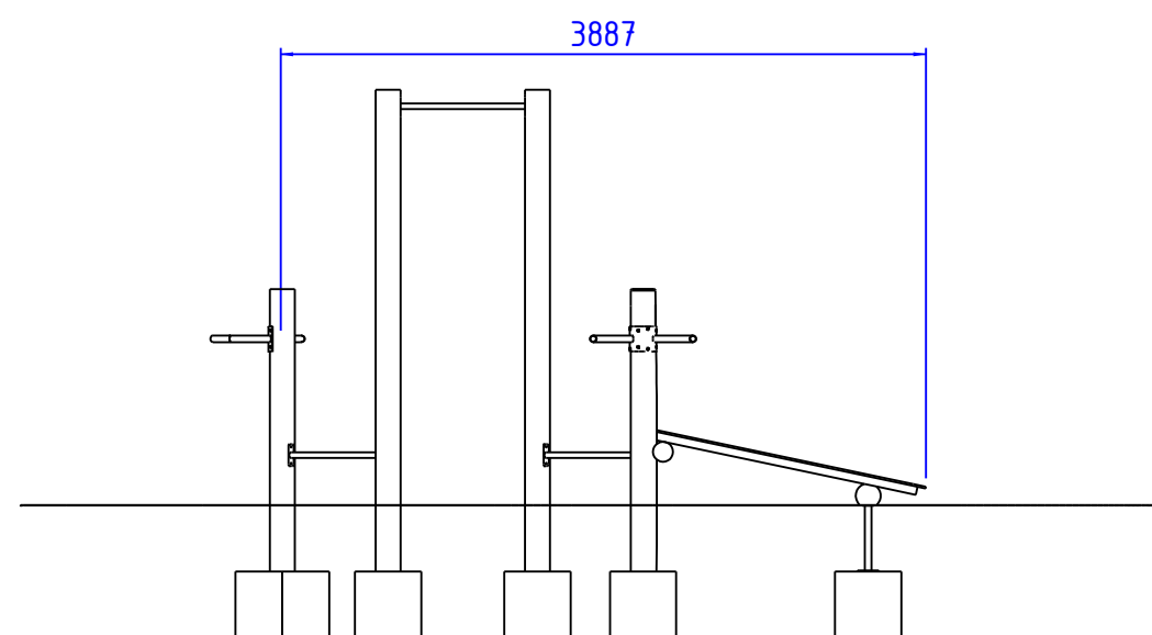
Vue côté
