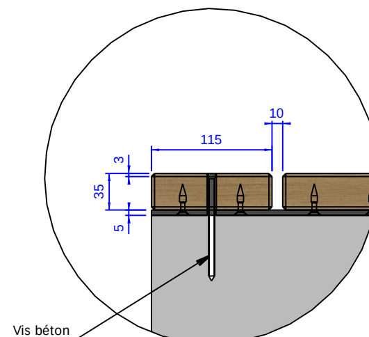
Fixation du module sur le banc en béton :
