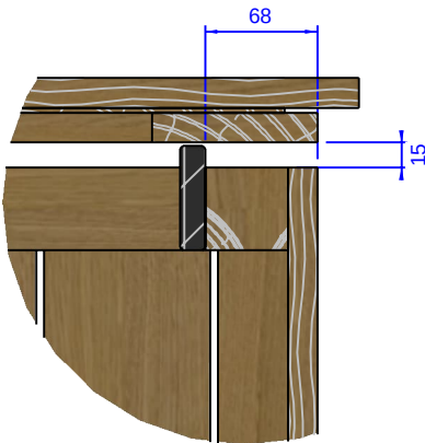
Système anti-pincement.
